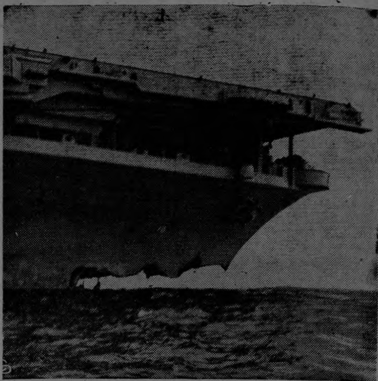
Esta foto, tomada desde una pequeña embarcación, muestra el boquete de 23 metros abierto en la proa del portaviones "Wasp" por el destructor "Hobson" cuando ambos barcos chocaron en el Atlántico. El Hobson se hundió inmediatamente. (INP)
